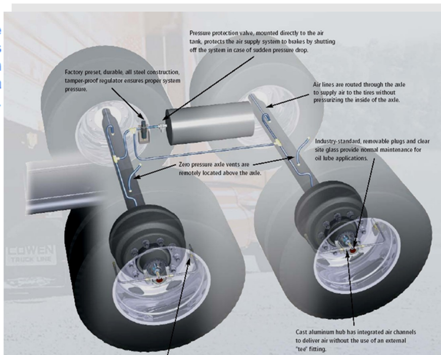
DETALLE DE TAPON MAZA
